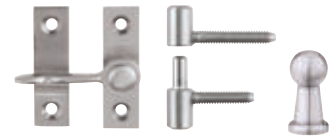
Draairaambeslagset RVS bestaat uit: • Tramklink (2x) • Paumelle (2x) • Raamknop (1x)
